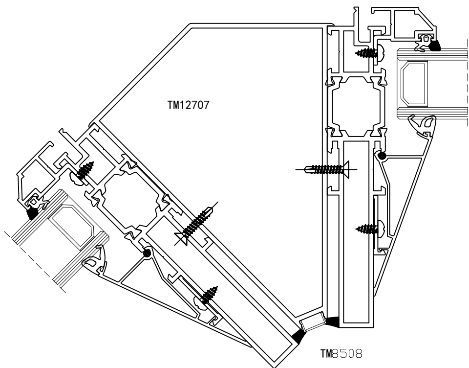
135° 转角料
