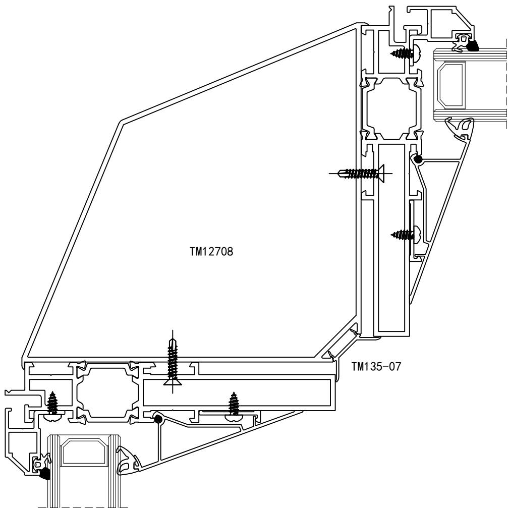
90° 转角料
