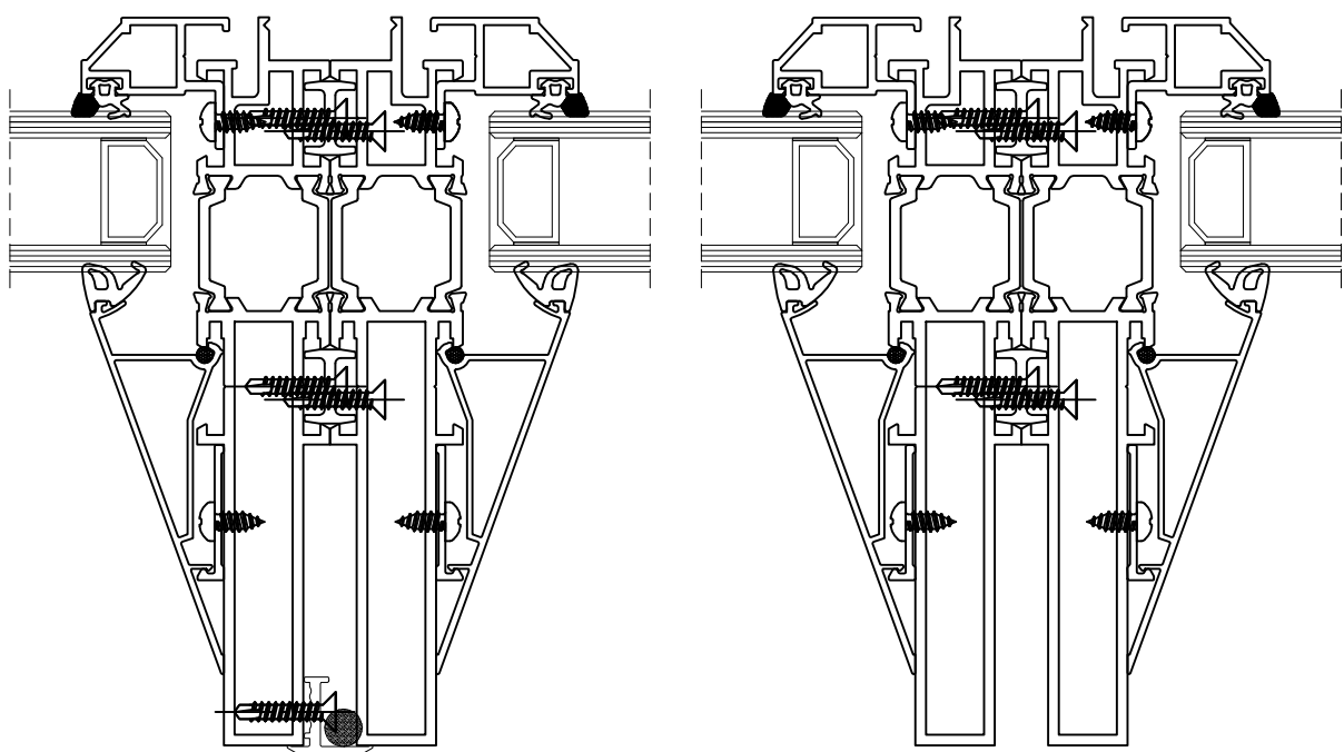
拼樘收口料
